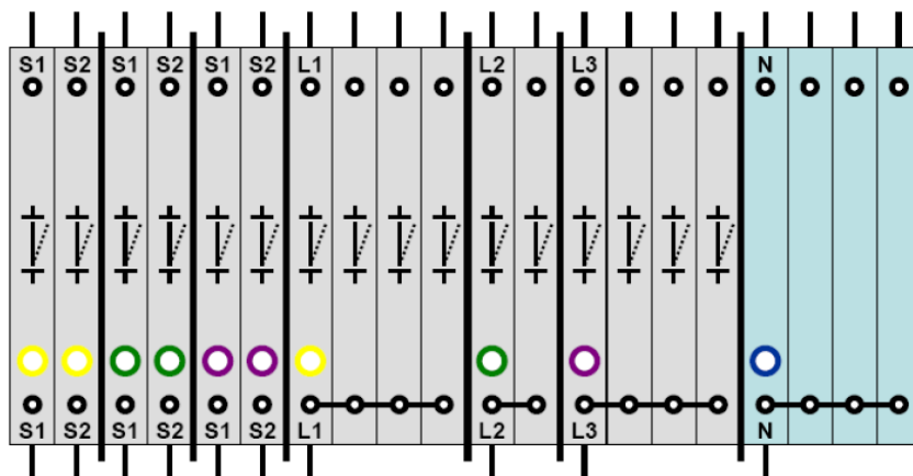
Abbildung 1: Aufbau der Prüf- und Steuerklemme
